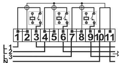
Slika 6. Šema vezivanja - direktna veza
